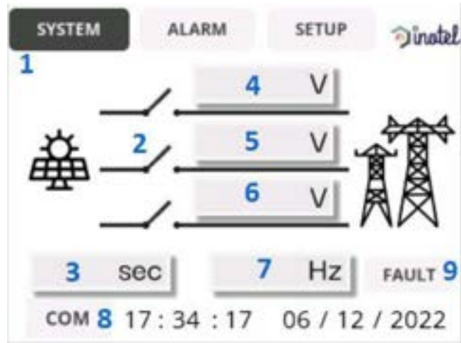
Resim 1: Sistem Ekranı
